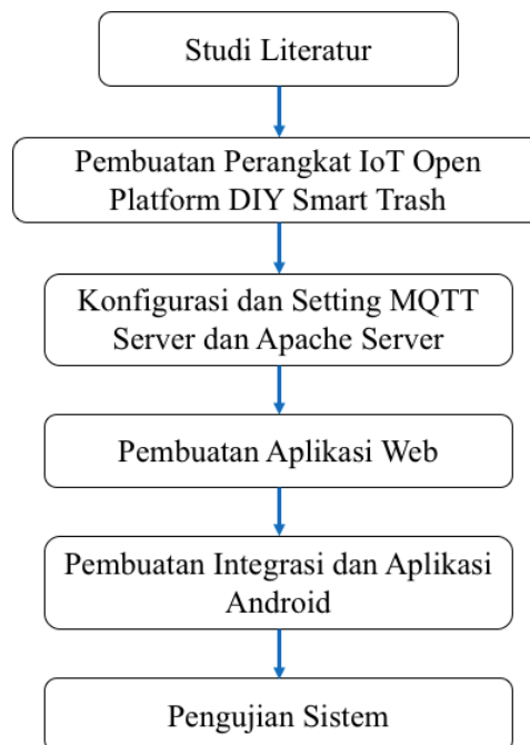
Gambar 4. Metodologi Penelitian
